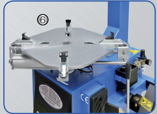
(1) Güçlü Lastik Presi (2) Profesyonel Kullanım için Destek Kolu (3) Montaj Kafası (4) Hassas Ayar İçin Joystick (5) Ayak Pedalları (6) Özel Çelik Tırnaklar 10" – 24"
