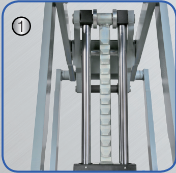
(1) Otomatik Kilitleme ve Kilit Açma Sistemi (2) Külbütör Makas Sistemi (3) Ultra Alçak Yapı
