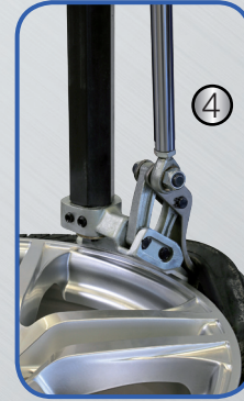
(1) Dinamik Lastik Sökme Ekipmanı (2) Otomatik, Havalı Jant Tırnağı (3) Kullanıcı Dostu Kontrol Ünitesi (4) Otomatik Montaj Kafası (5) Kolay Lastik Yerleştirme
