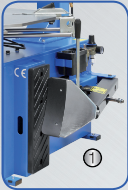
(1) Güçlü Lastik Presi (2) Profesyonel Kullanım için Destek Kolu (3) Montaj Kafası (4) Hassas Ayar İçin Joystick (5) Ayak Pedalları (6) Özel Çelik Tırnaklar 10" – 24"
